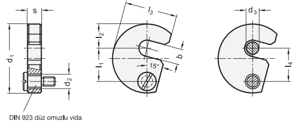
DIN 923 düz omuzlu vida
